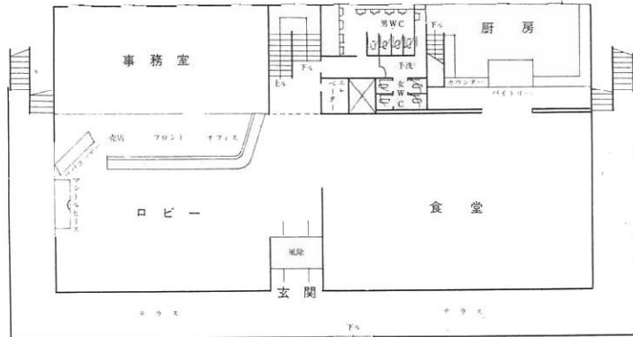
本館2階平面図
