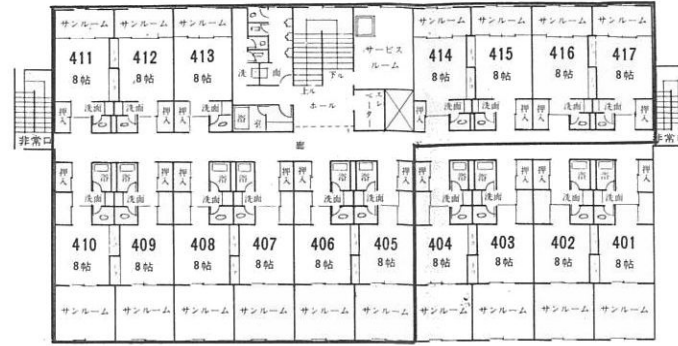
本館4階平面図
