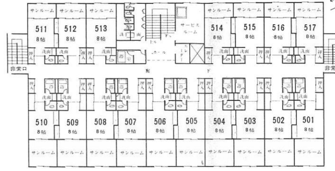
本館5階平面図
