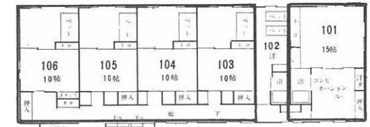
第2新館1階平面図
